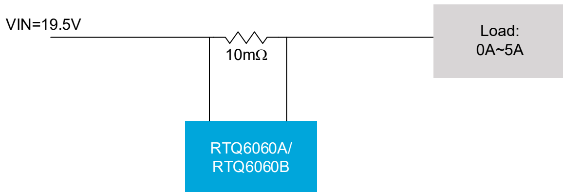
圖6. RTQ6060A 和 RTQ6060B 應用於桌上型電腦
