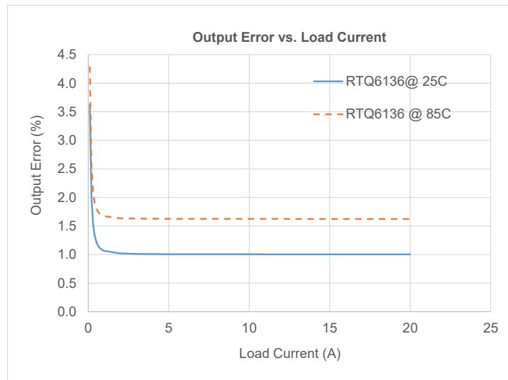
圖 9. RTQ6136 誤差評估曲線
