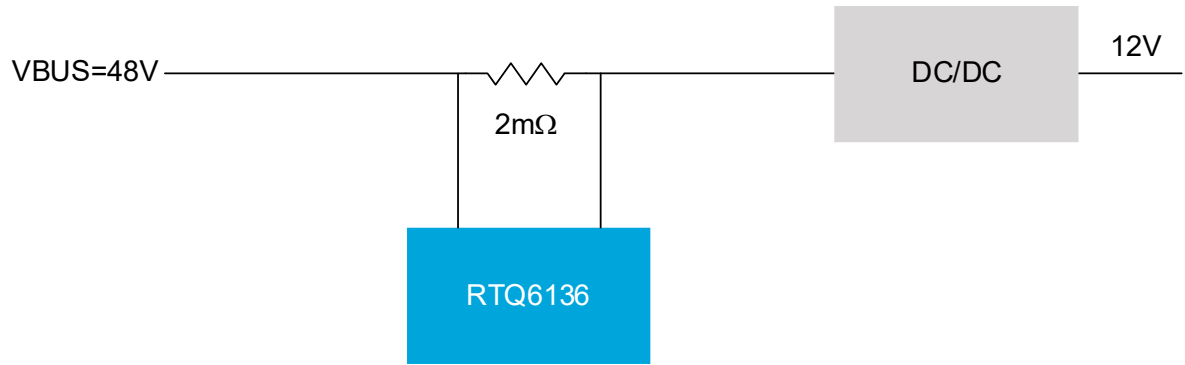
圖 8. RTQ6136 應用於伺服器
