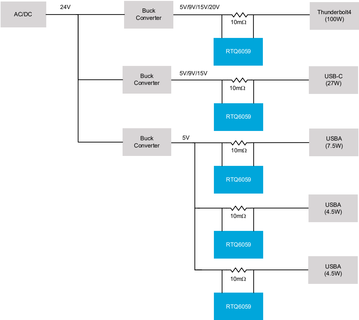
圖4. RTQ6059 應用於USB系統
