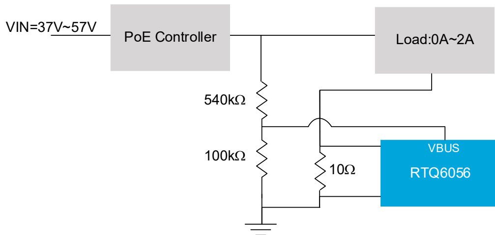
圖2. RTQ6056 應用於 PoE 系統
