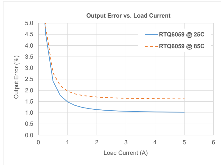
圖5. RTQ6059 誤差評估曲線
