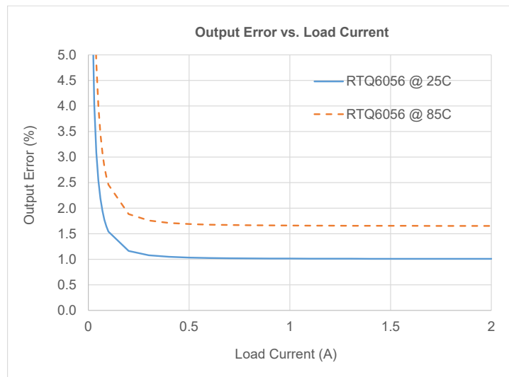
圖3. RTQ6056 誤差評估曲線
