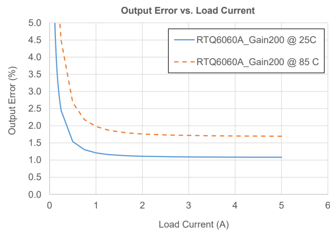
圖7. RTQ6060A 誤差評估曲線
